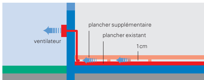
Ventilation d'un double plancher dans un local
